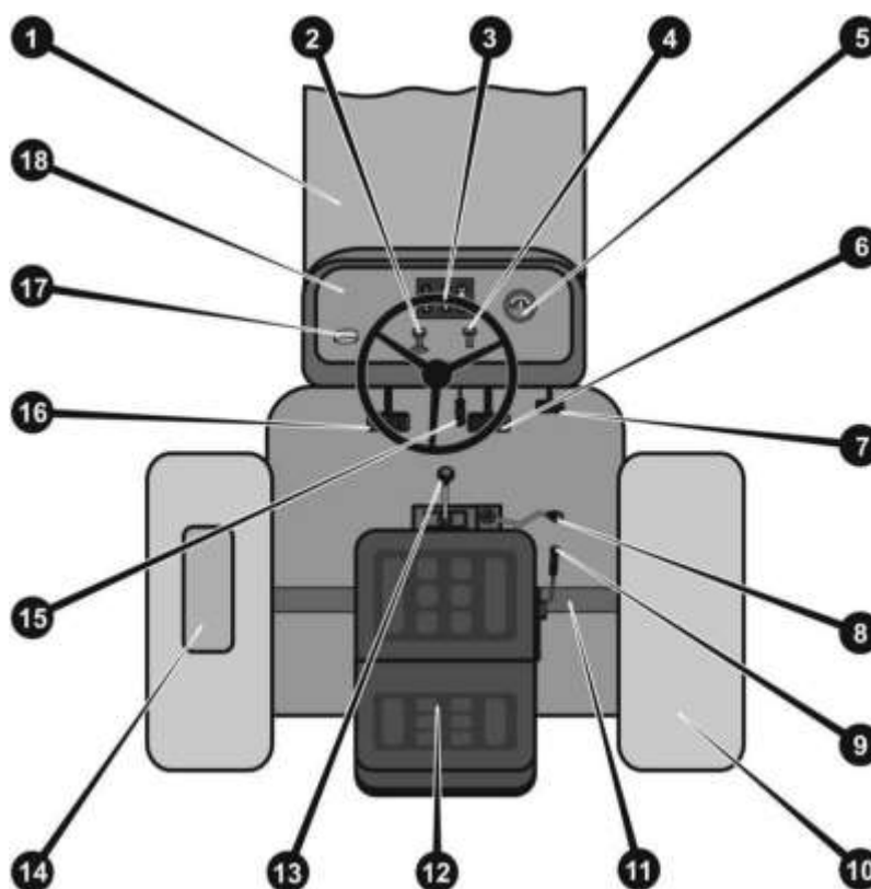
Рисунок 3.2. Схема расположения органов управления трактора
