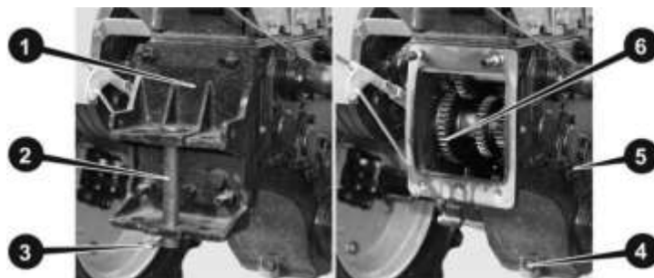
Рисунок 4.1. Прицепная цапфа.
