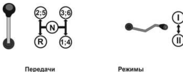
Рисунок 3.9. Переключение передач и режимов Трактора малогабаритного РУСИЧ модель Т-15 (15л.с.)
