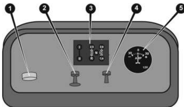
Рисунок 3.7. Панель приборов
